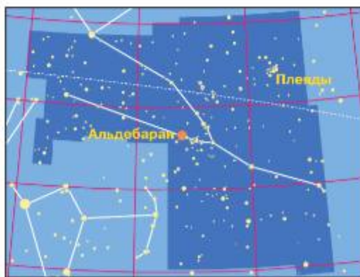
Созвездие Телец
