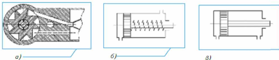
Рис. 4.3. Схемы работы пневматического двигателя: а — турбинного; б — цилиндрического с односторонней подачей воздуха; в — цилиндрического с двухсторонней подачей воздуха
