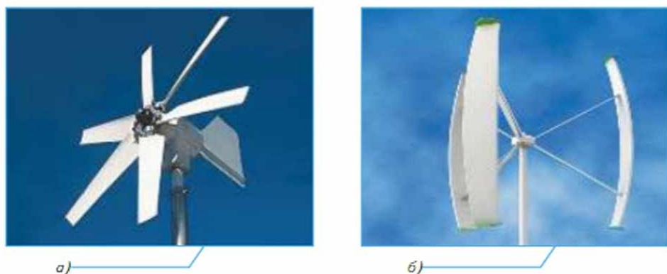
Рис. 4.2. Ветровые двигатели малой и средней мощности: а — с горизонтальной осью по схеме пропеллера; б — с вертикальной осью с лопатками
